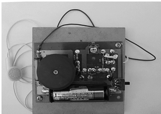
完成ラジオです
